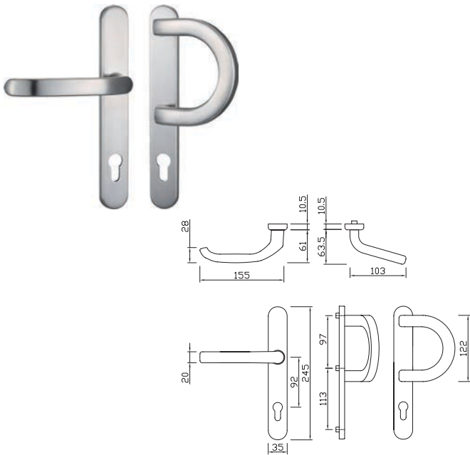
DG 58.ER.SSWB PZ 92 Door Handle
