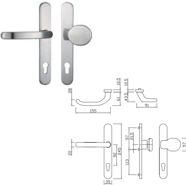
DG 58.ER.SSWK PZ 92 Door Handle
